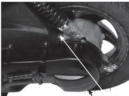
Aftapningsskrue Påfyldningsskrue
